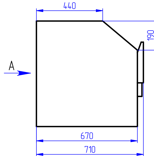
Вид А
